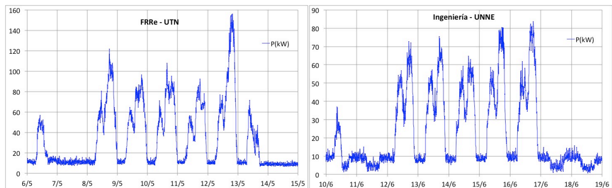
Figura 1: Curvas de demanda de Potencia Activa [kW] correspondientes a la Facultad Regional Resistencia de la UTN y a la Facultad de Ingeniería de la UNNE
